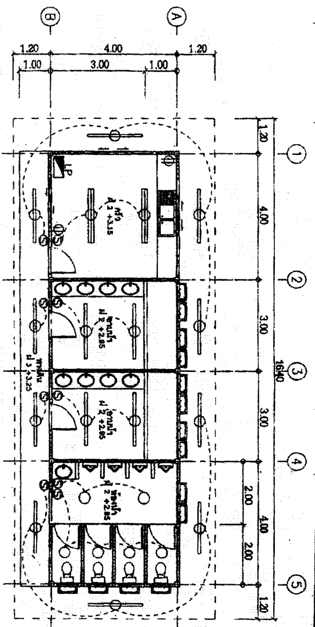
Коллекторный зал 1:20
